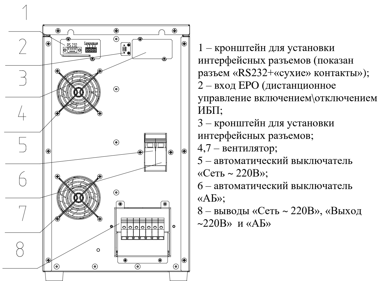
Рисунок 1.2 – ИБП Штиль ST1106L, ST1110L. Вид с тыльной стороны
